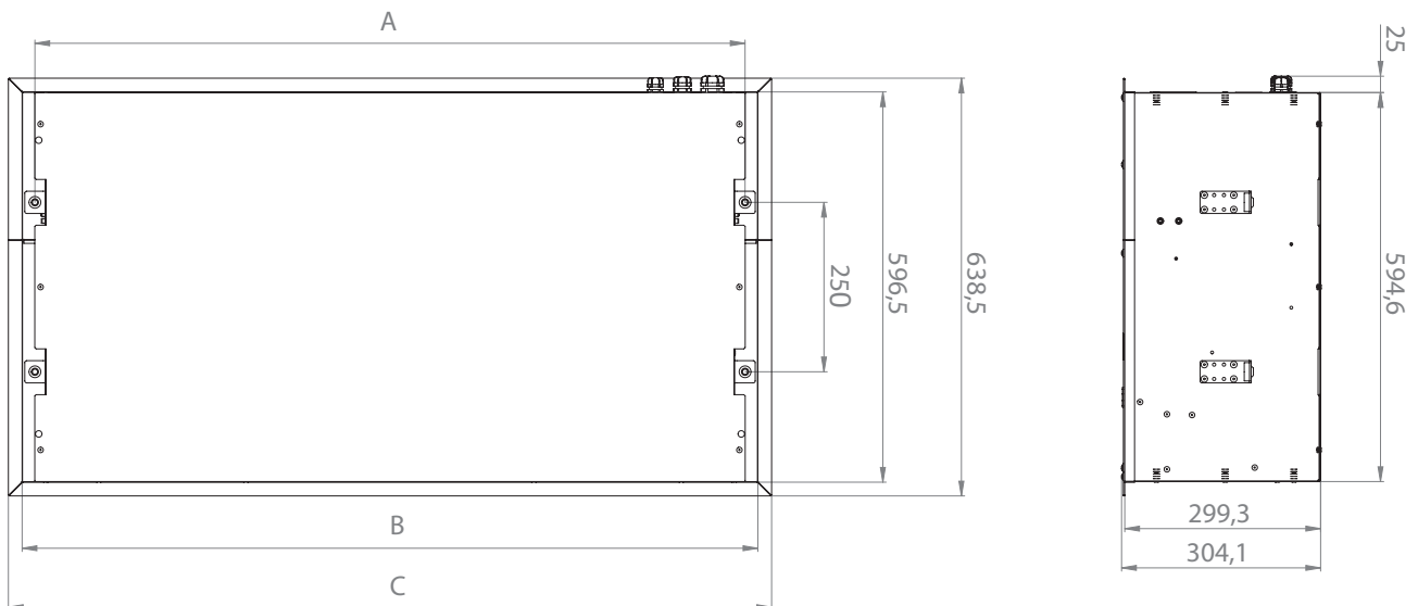
Air curtain dimensions Abmessungen des Luftschleiers
